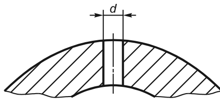
Диаметр d — 3,2 мм с допуском \pm 0,1 мм
